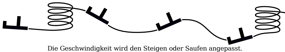
Luftmassenbewegung
